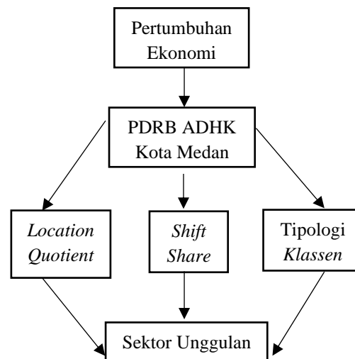
Gambar. 2 Kerangka Konseptual
